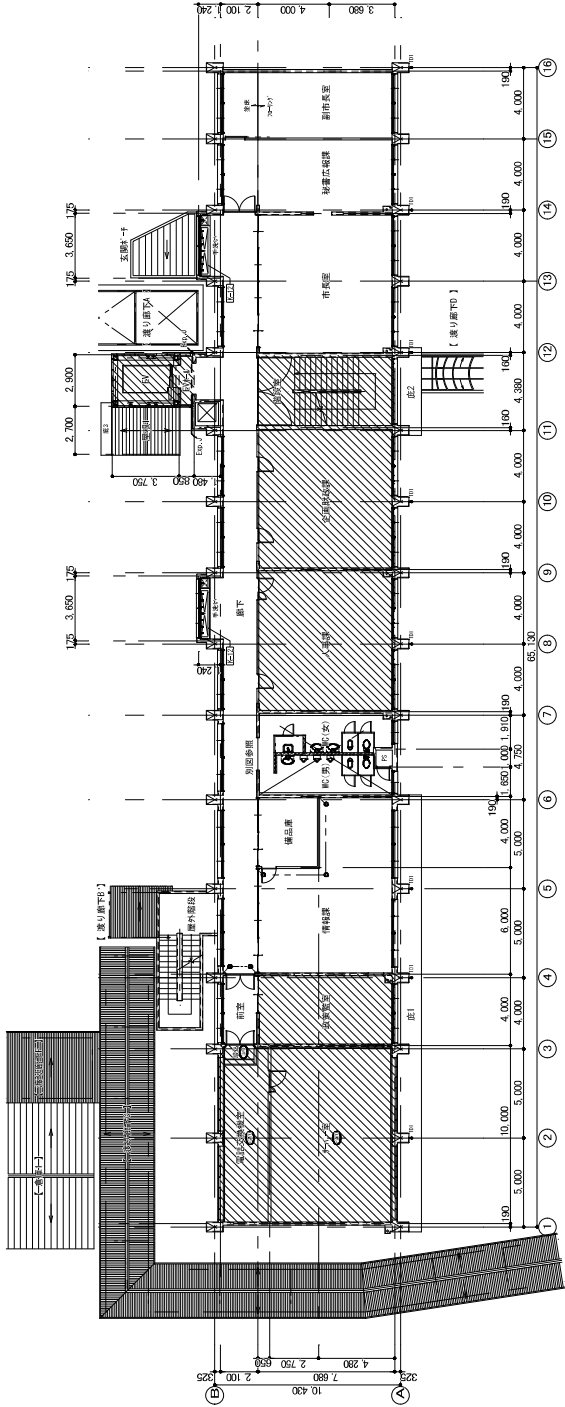
改修前：2階平面図
