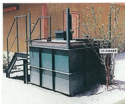
小型メタンガス発生装置
