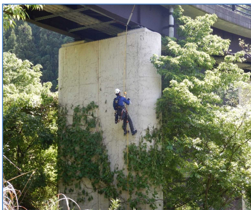
【ロープアクセスによる点検状況】
